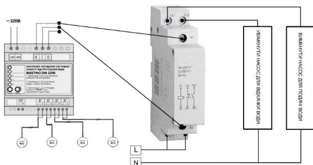
Схема підключення контролера Mastino DIN 220B до насоса
